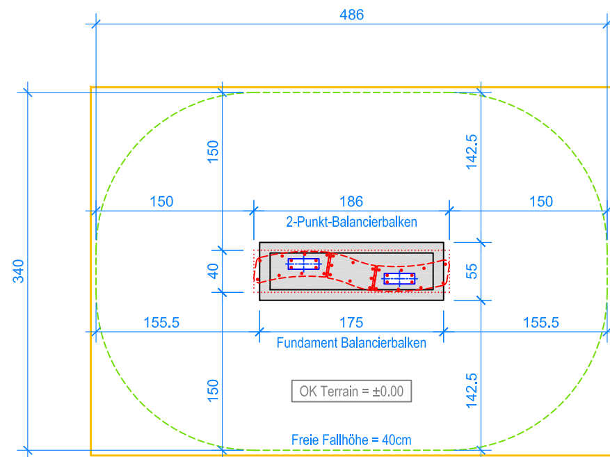
GRUNDRISS 1:50
