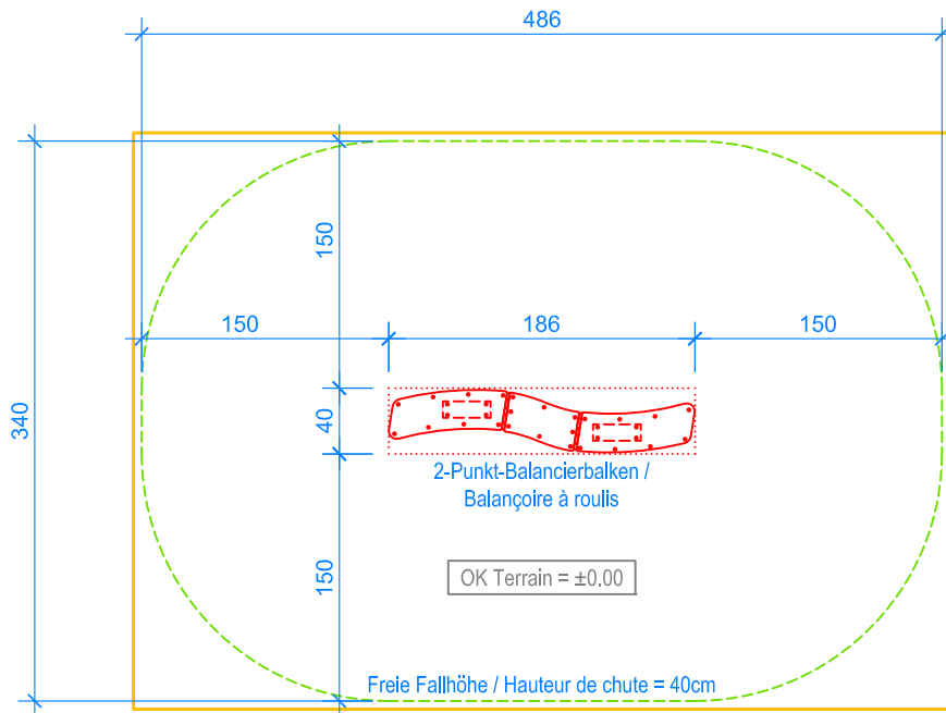
GRUNDRISS / PLAN 1:50
