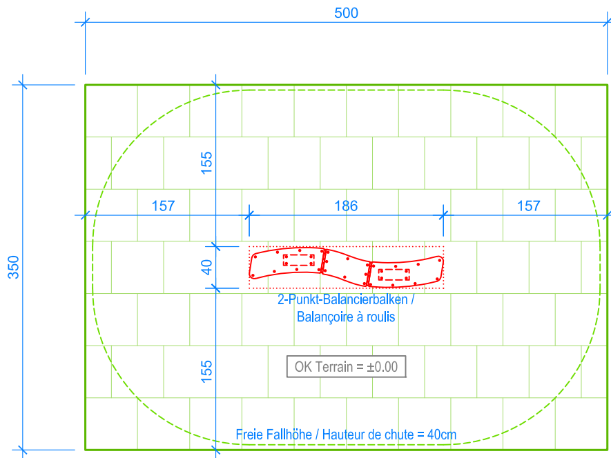
GRUNDRISS / PLAN 1:50
