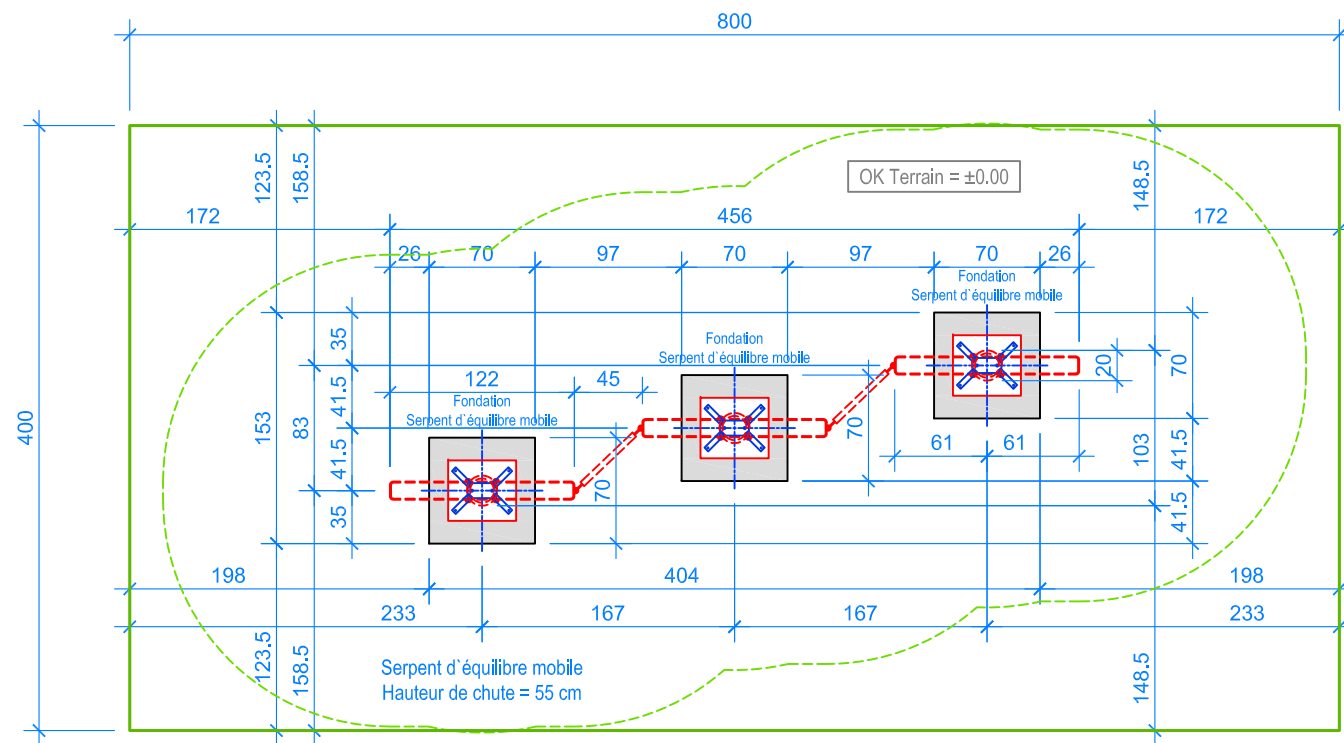
PLAN 1:50
