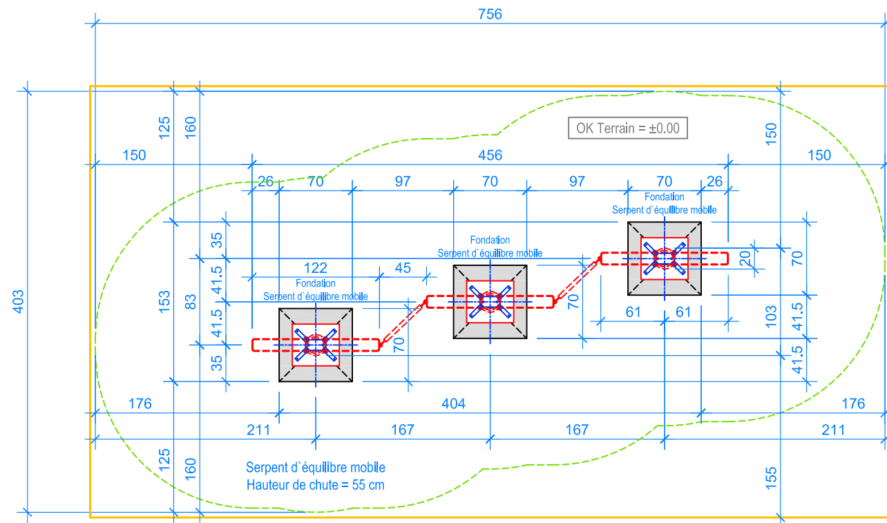
PLAN 1:50
