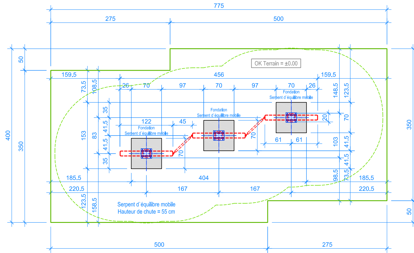
PLAN 1:50
