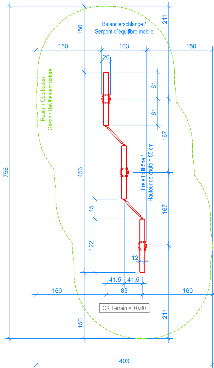
GRUNDRISS / PLAN 1:50
