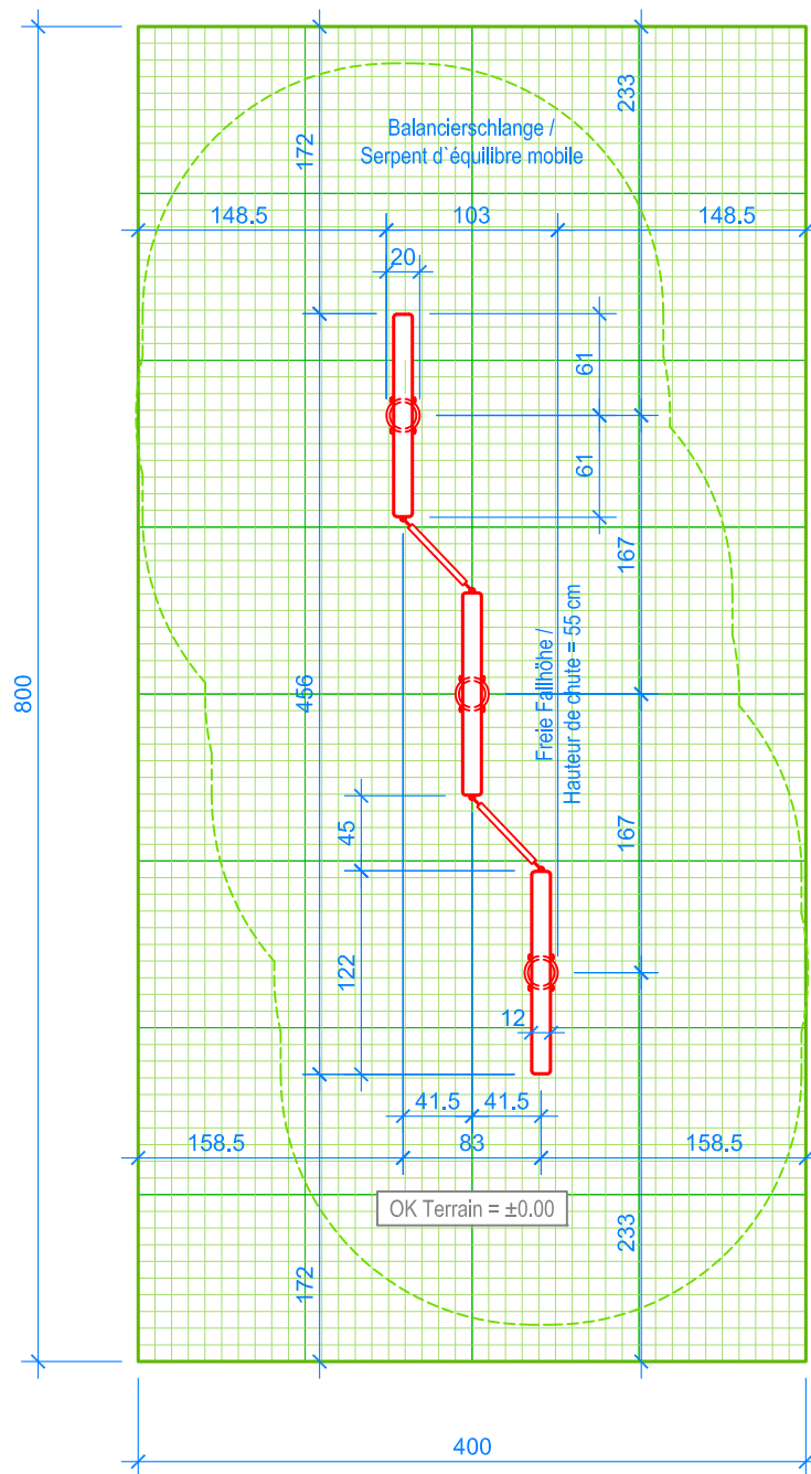
GRUNDRISS / PLAN 1:50
