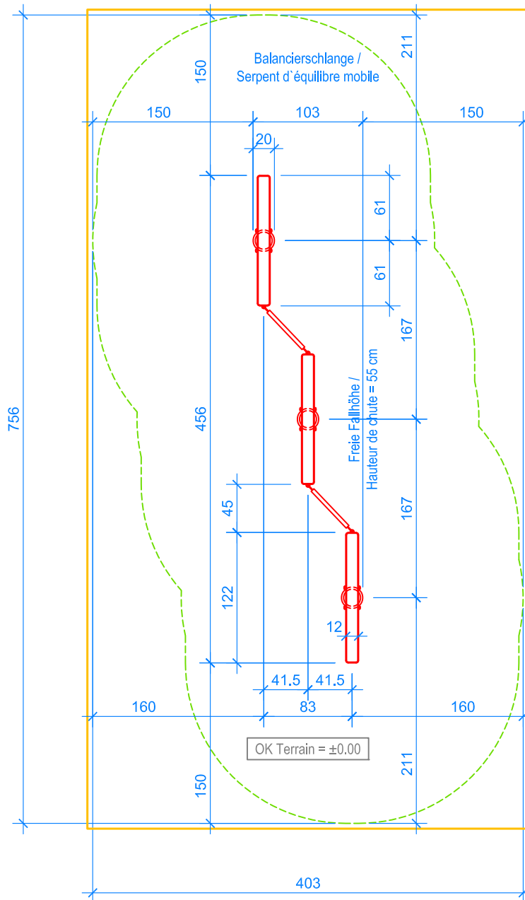
GRUNDRISS / PLAN 1:50
