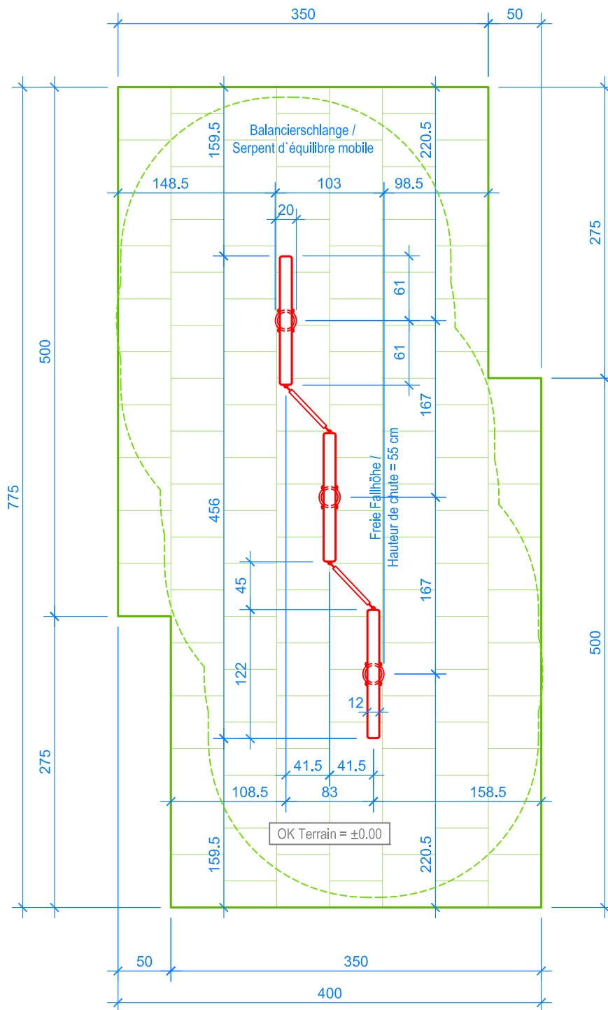
GRUNDRISS / PLAN 1:50
