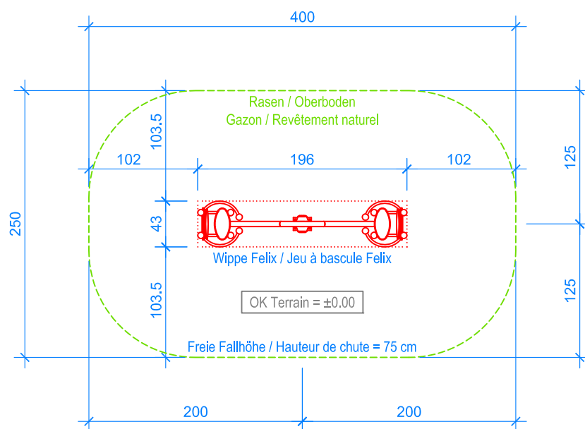
GRUNDRISS / PLAN 1:50
