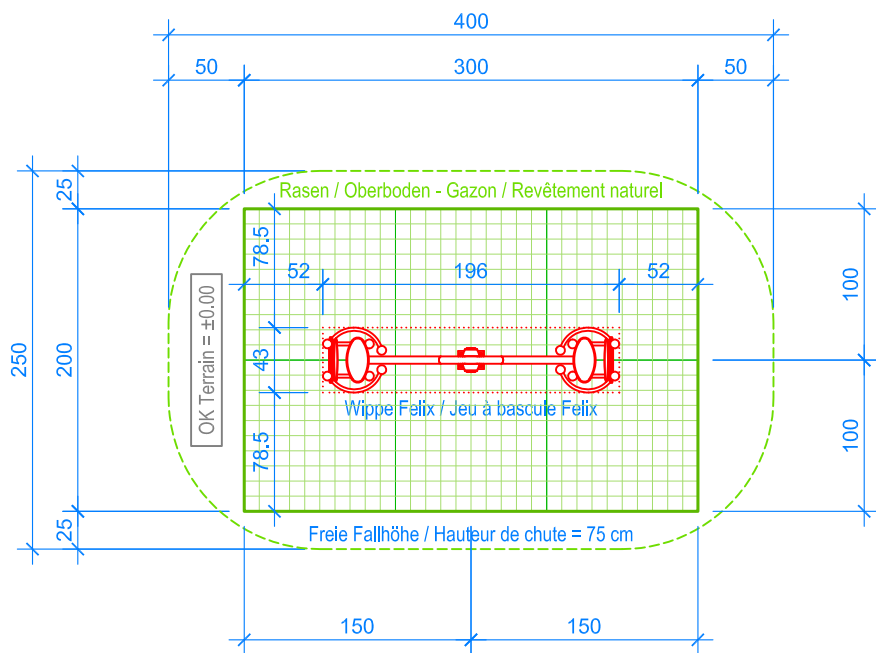
GRUNDRISS / PLAN 1:50
