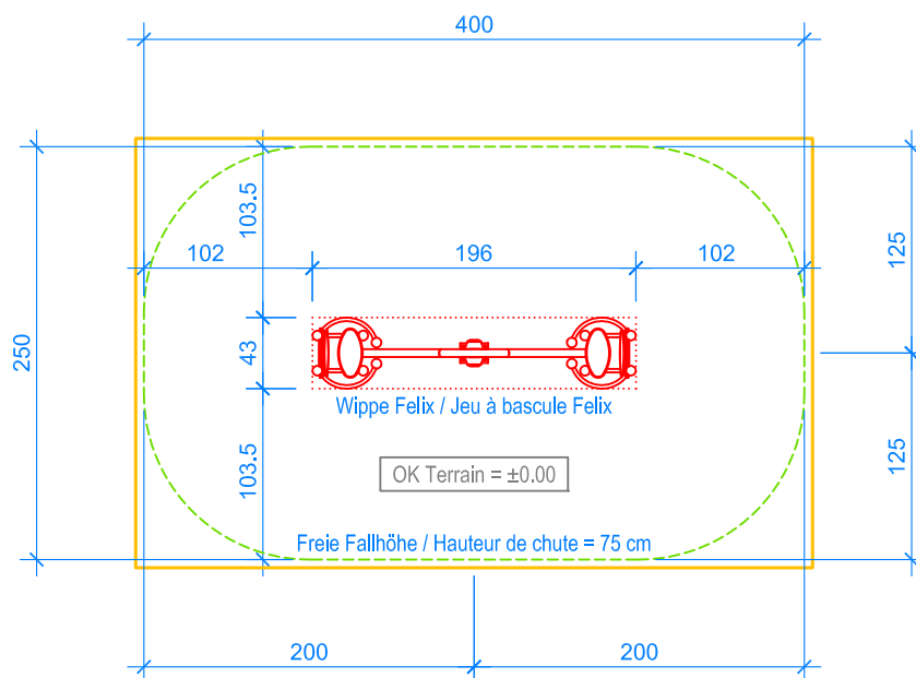
GRUNDRISS / PLAN 1:50
