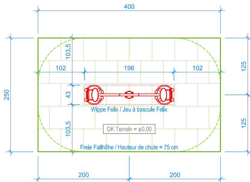
GRUNDRISS / PLAN 1:50
