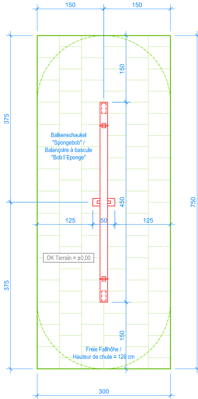
GRUNDRISS / PLAN 1:50
