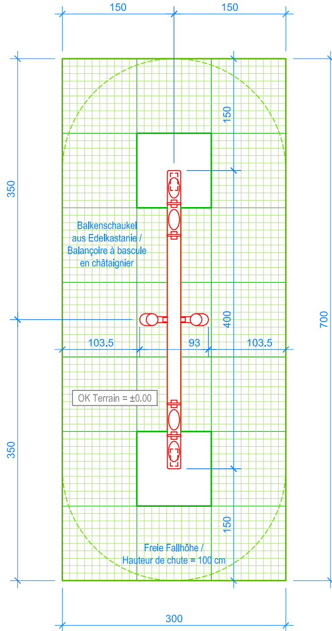
GRUNDRISS / PLAN 1:50
