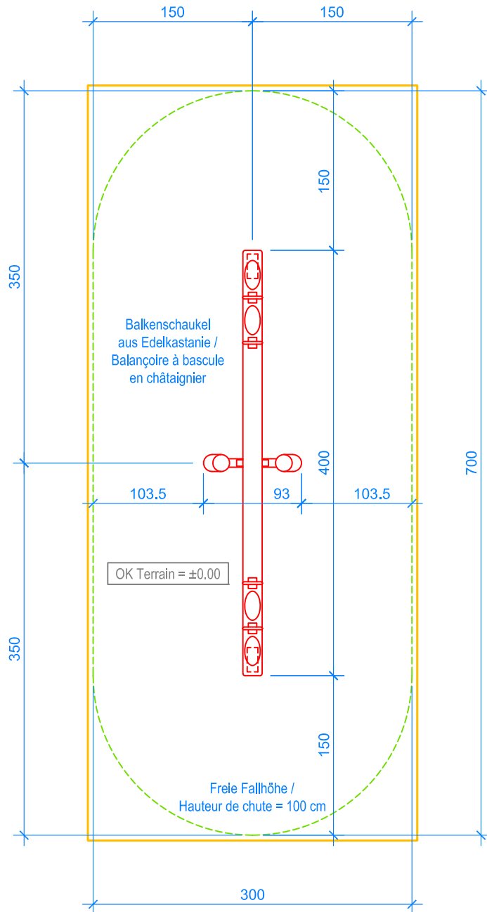
GRUNDRISS / PLAN 1:50
