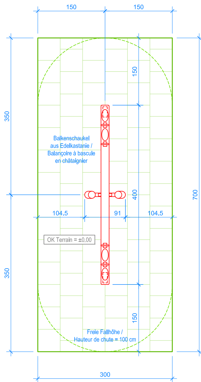
GRUNDRISS / PLAN 1:50
