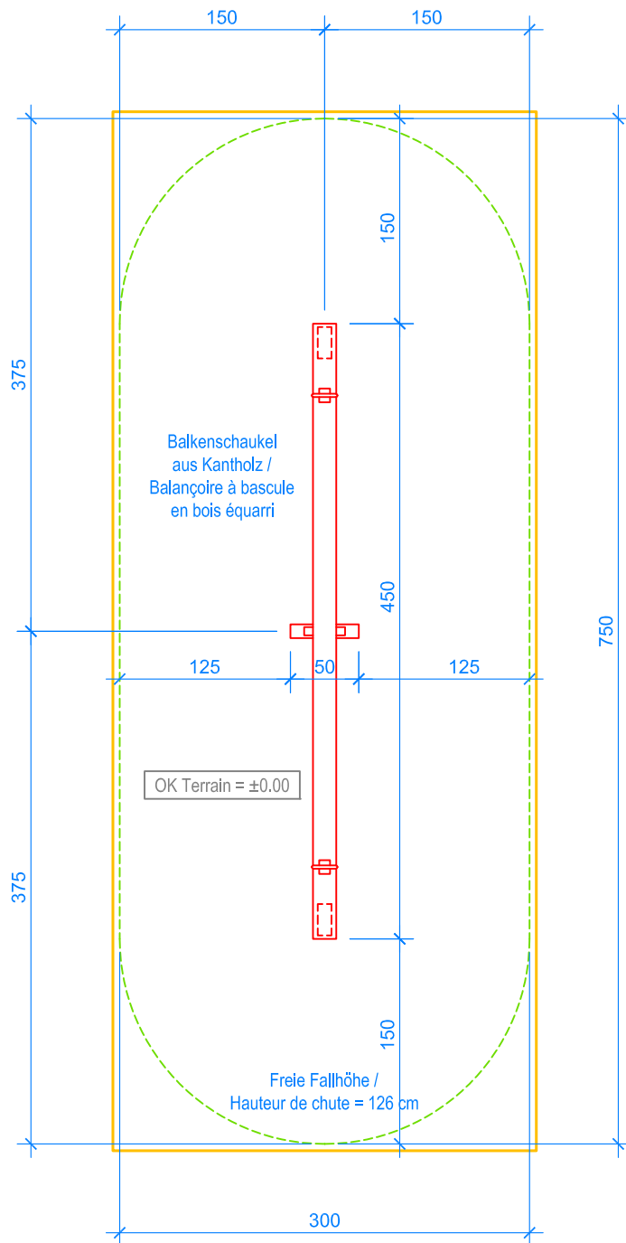
GRUNDRISS / PLAN 1:50
