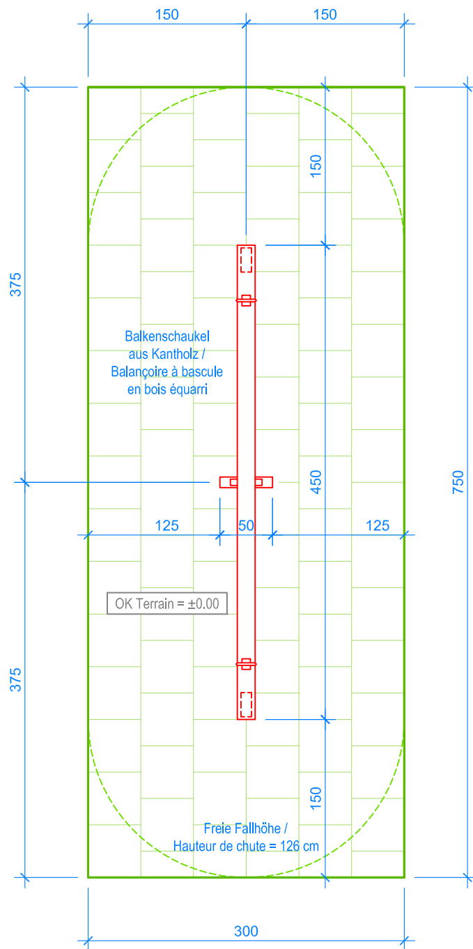
GRUNDRISS / PLAN 1:50
