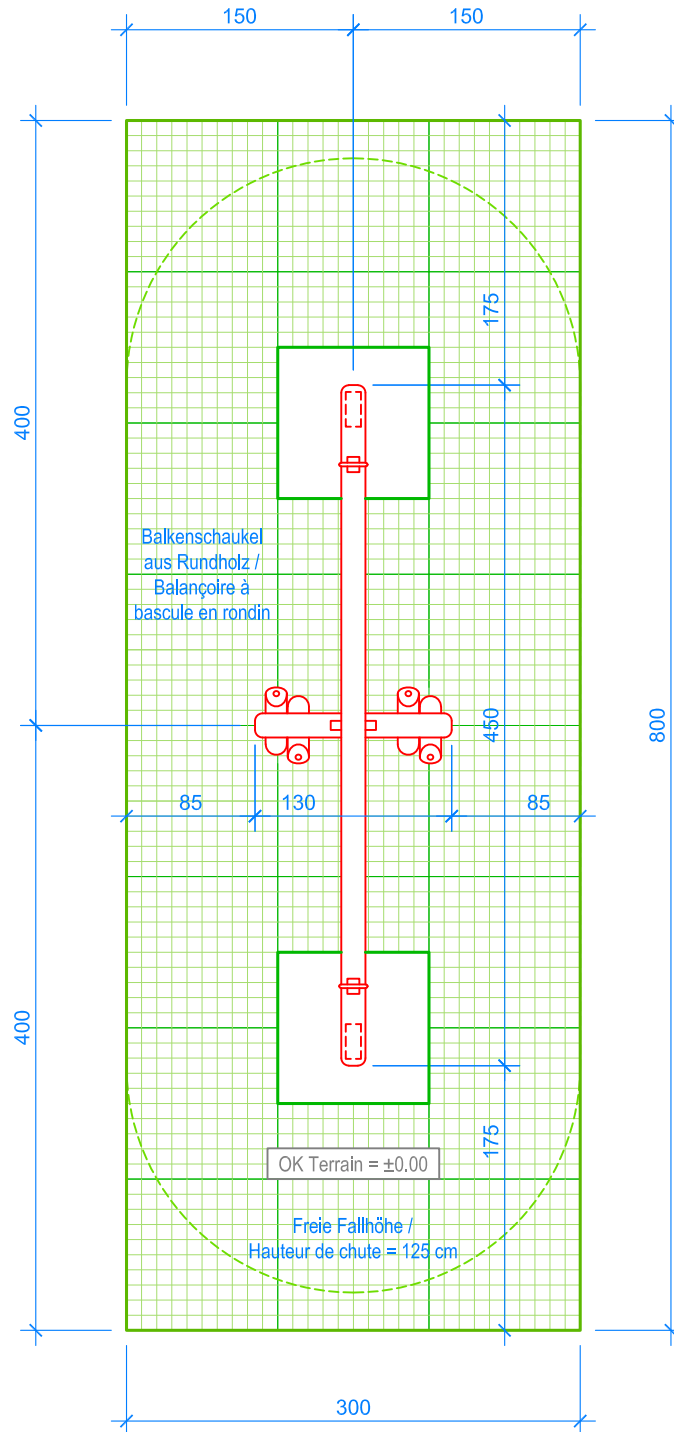
GRUNDRISS / PLAN 1:50
