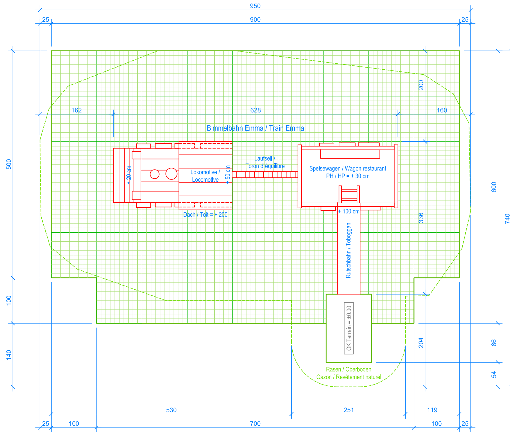
GRUNDRISS / PLAN 1:50
