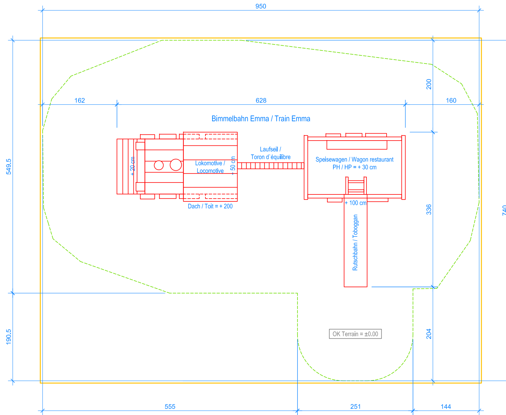
GRUNDRISS / PLAN 1:50
