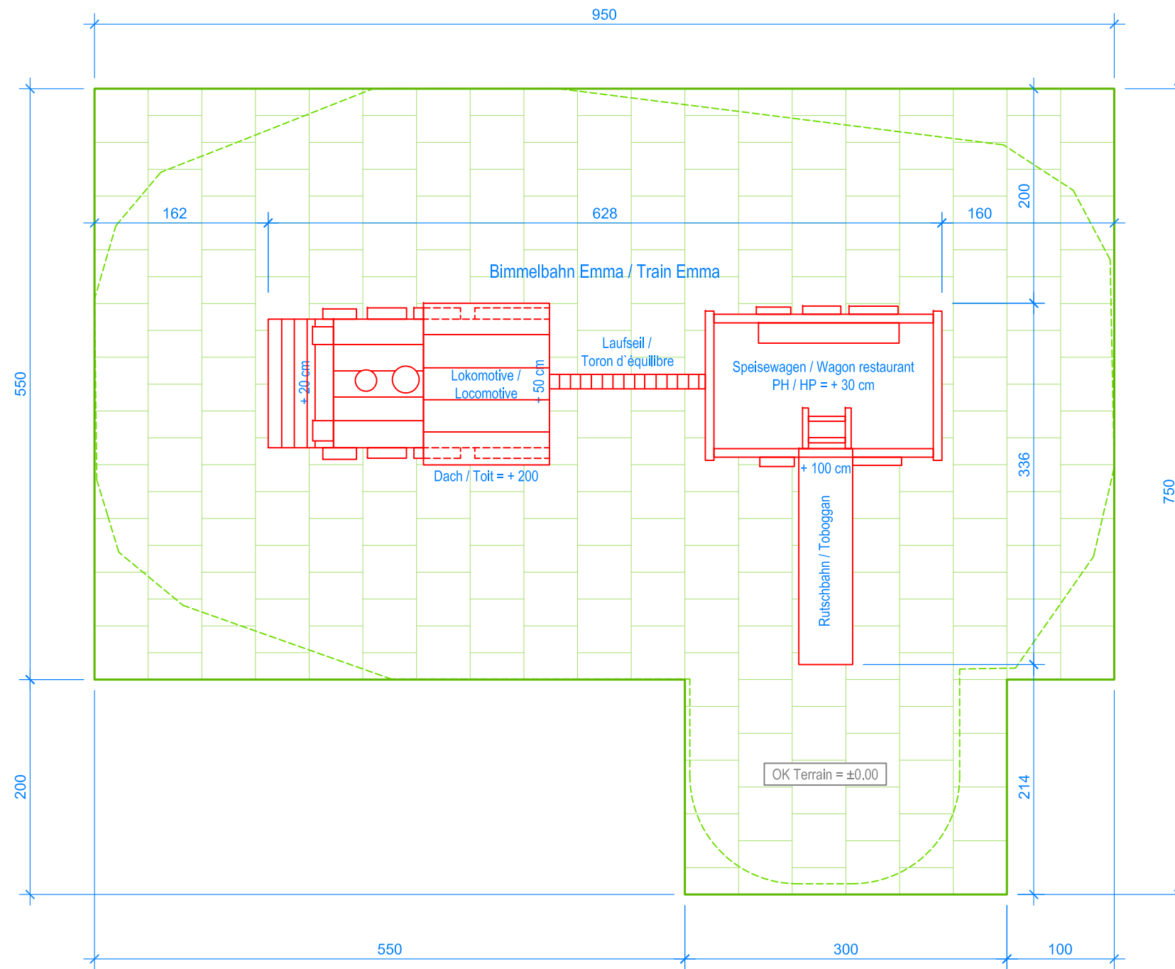
GRUNDRISS / PLAN 1:50
