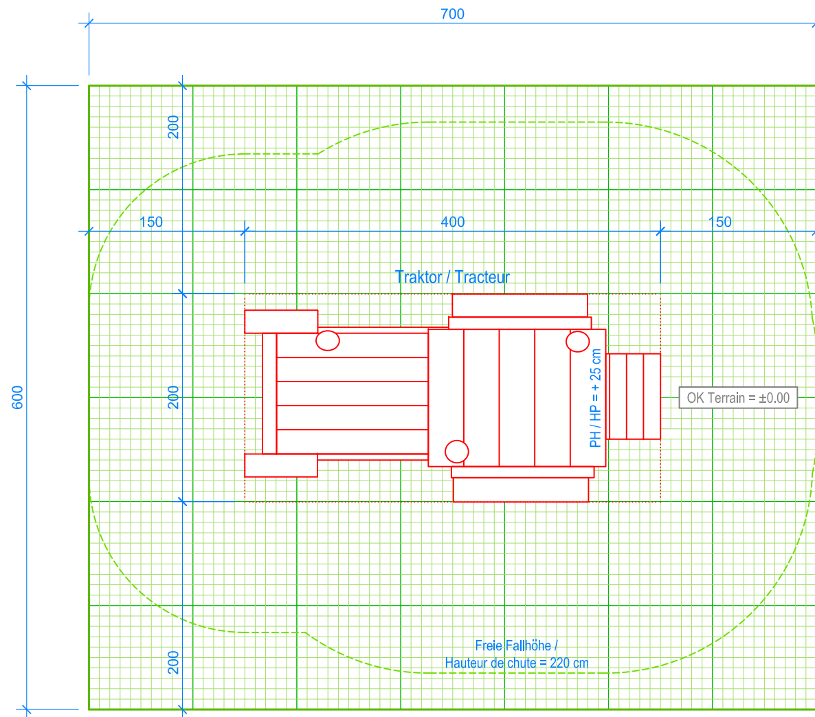
GRUNDRISS / PLAN 1:50
