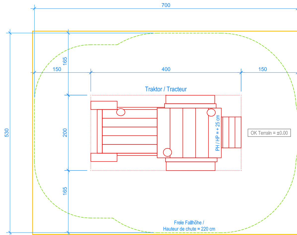
GRUNDRISS / PLAN 1:50
