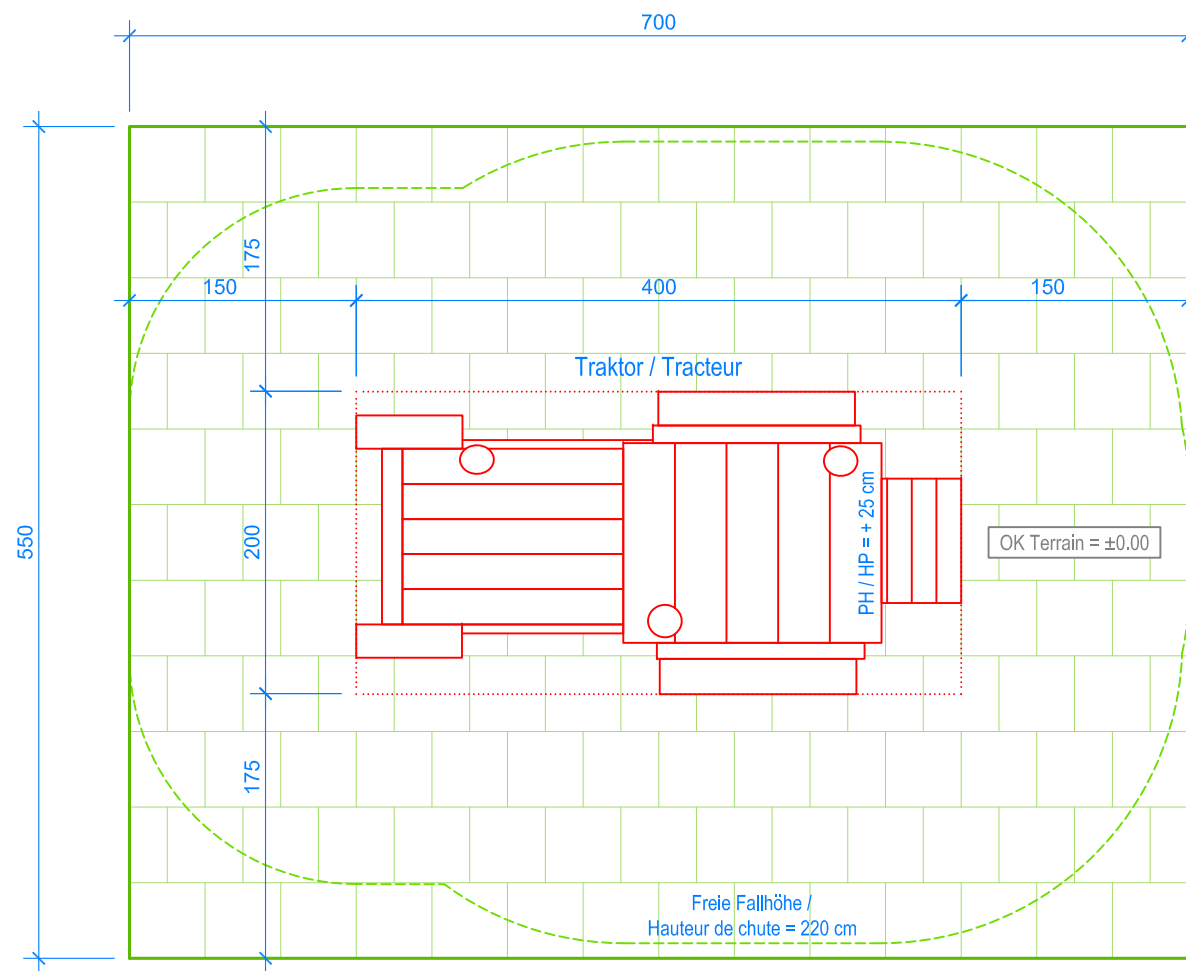
GRUNDRISS / PLAN 1:50
