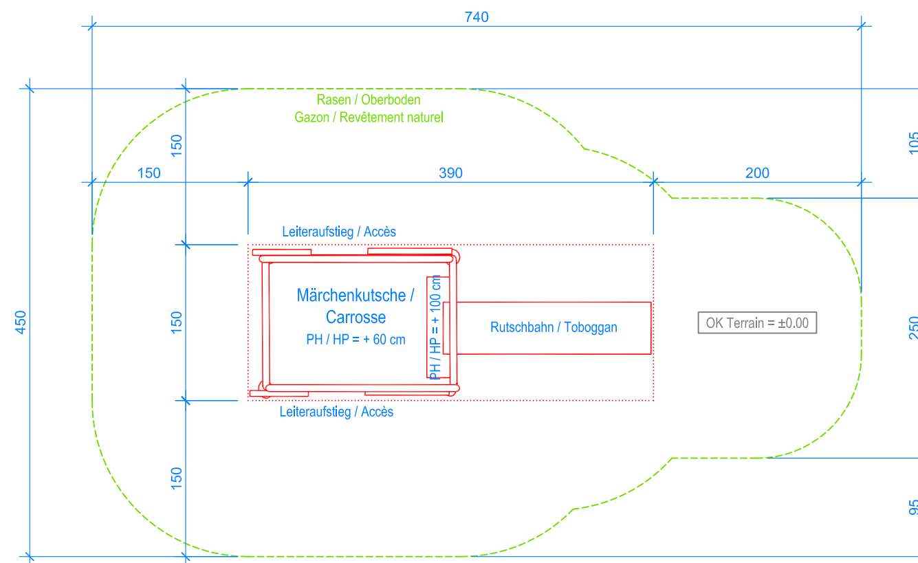
GRUNDRISS / PLAN 1:50
