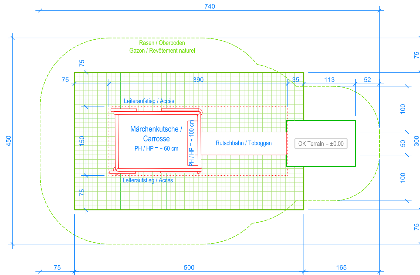
GRUNDRISS / PLAN 1:50
