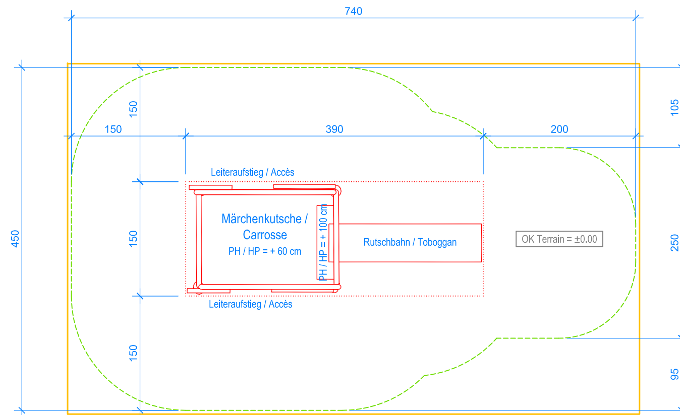
GRUNDRISS / PLAN 1:50
