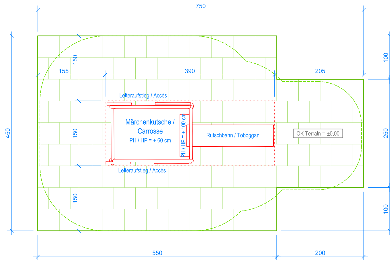
GRUNDRISS / PLAN 1:50
