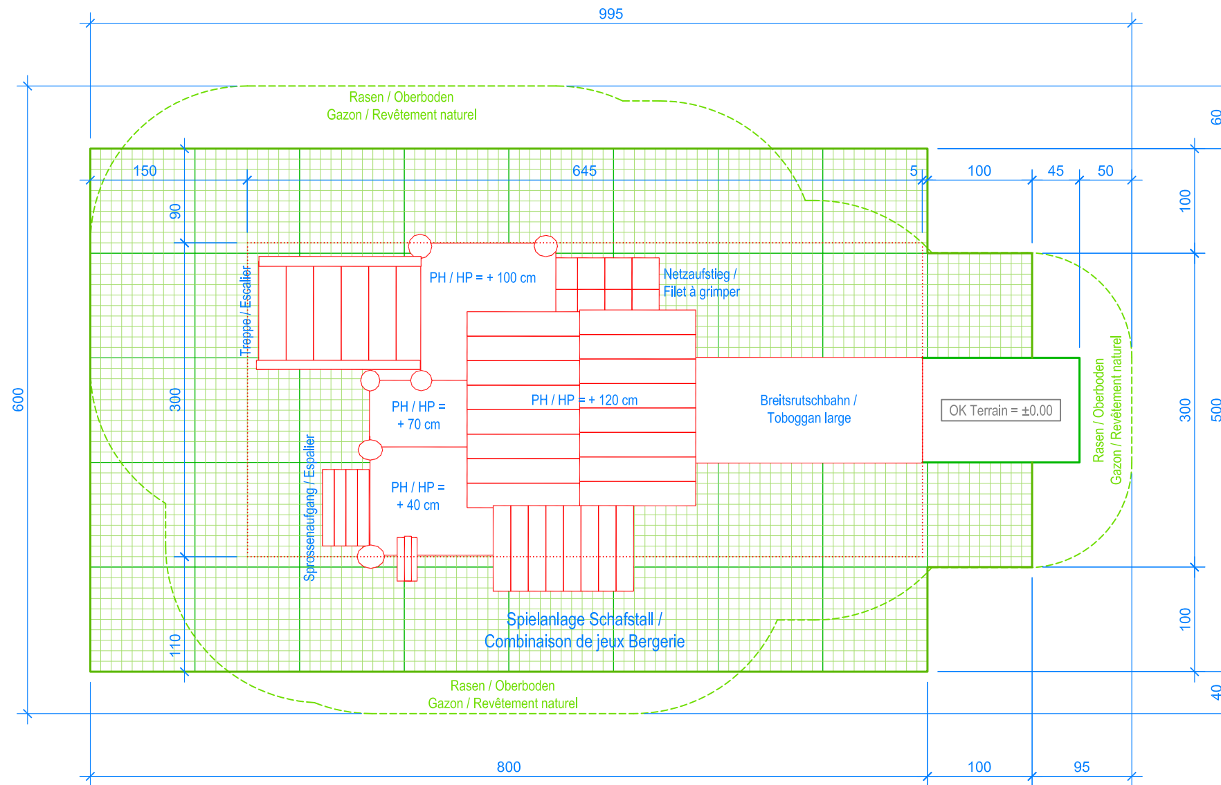
GRUNDRISS / PLAN 1:50
