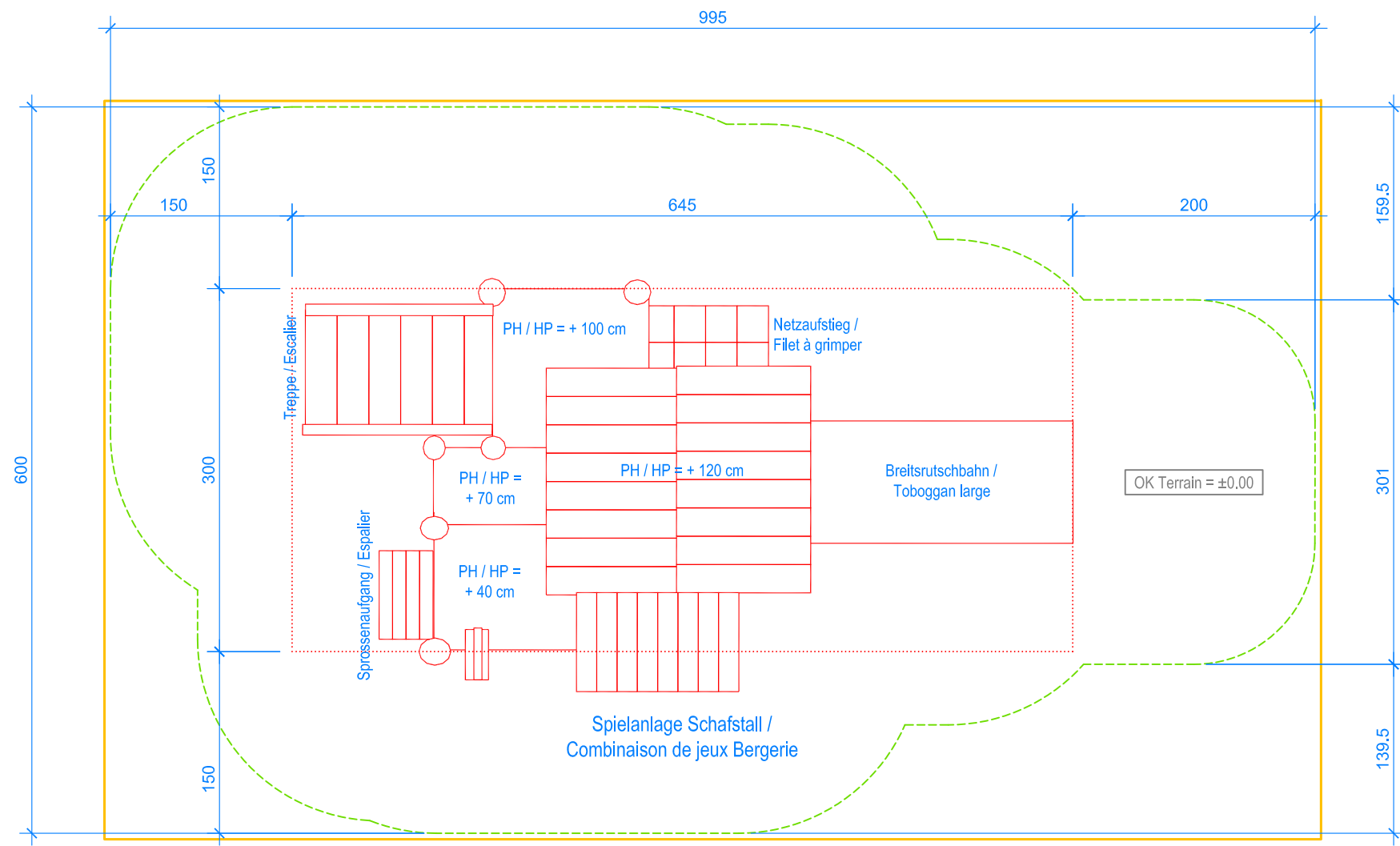
GRUNDRISS / PLAN 1:50
