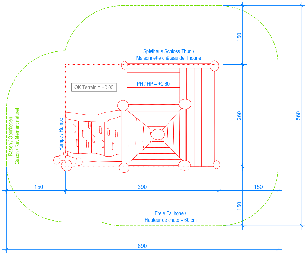
GRUNDRISS / PLAN 1:50
