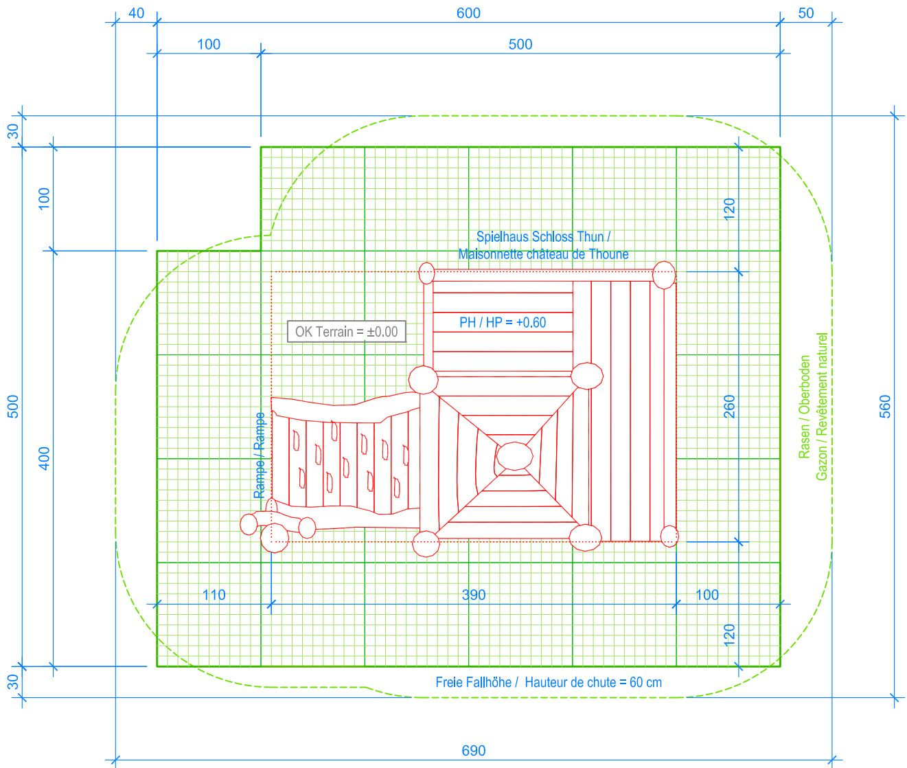
GRUNDRISS / PLAN 1:50
