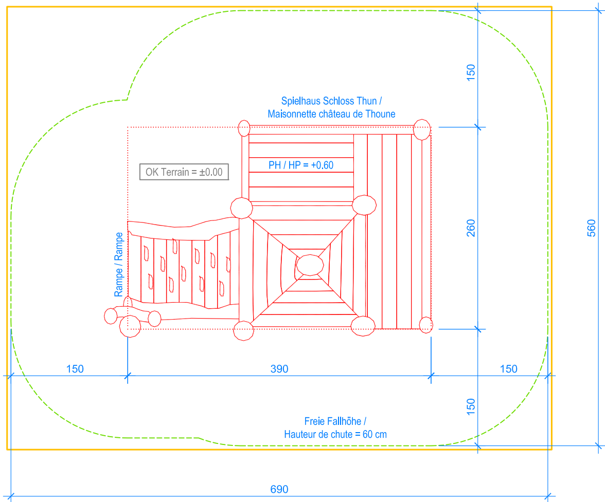
GRUNDRISS / PLAN 1:50
