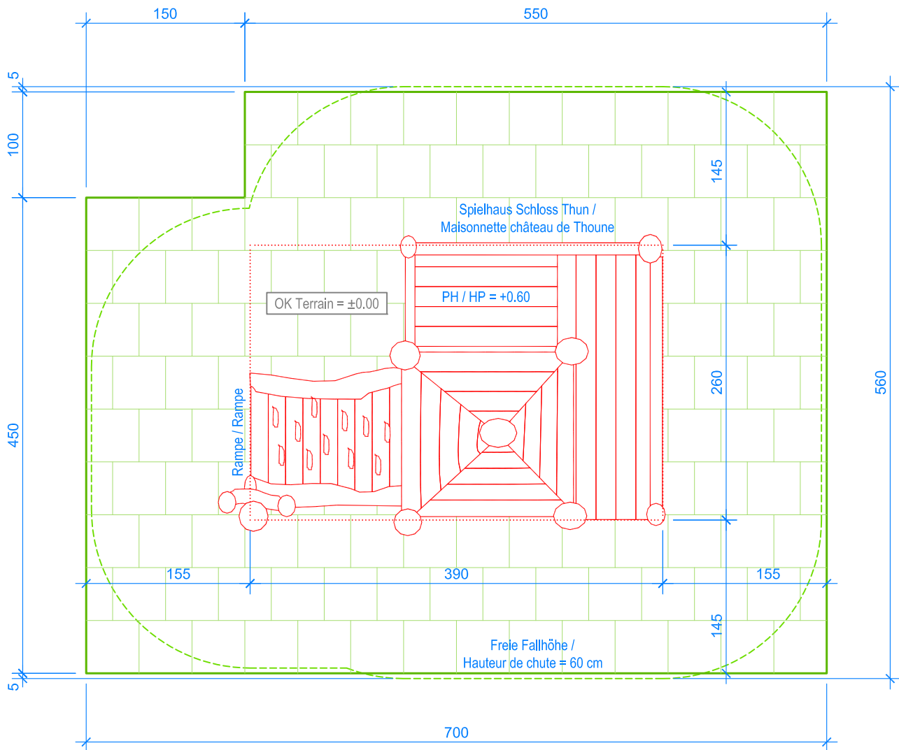
GRUNDRISS / PLAN 1:50
