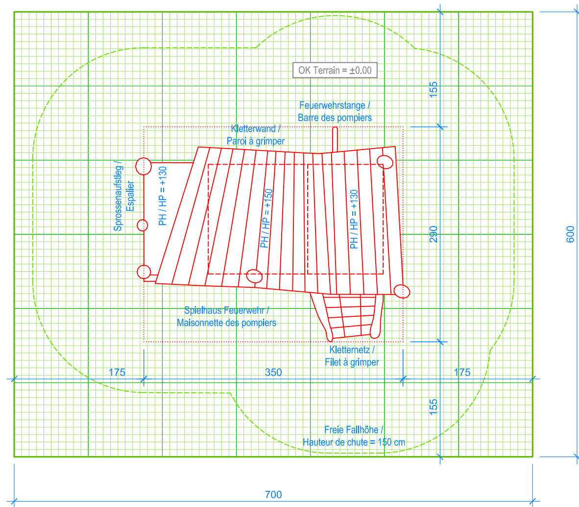
GRUNDRISS / PLAN 1:50
