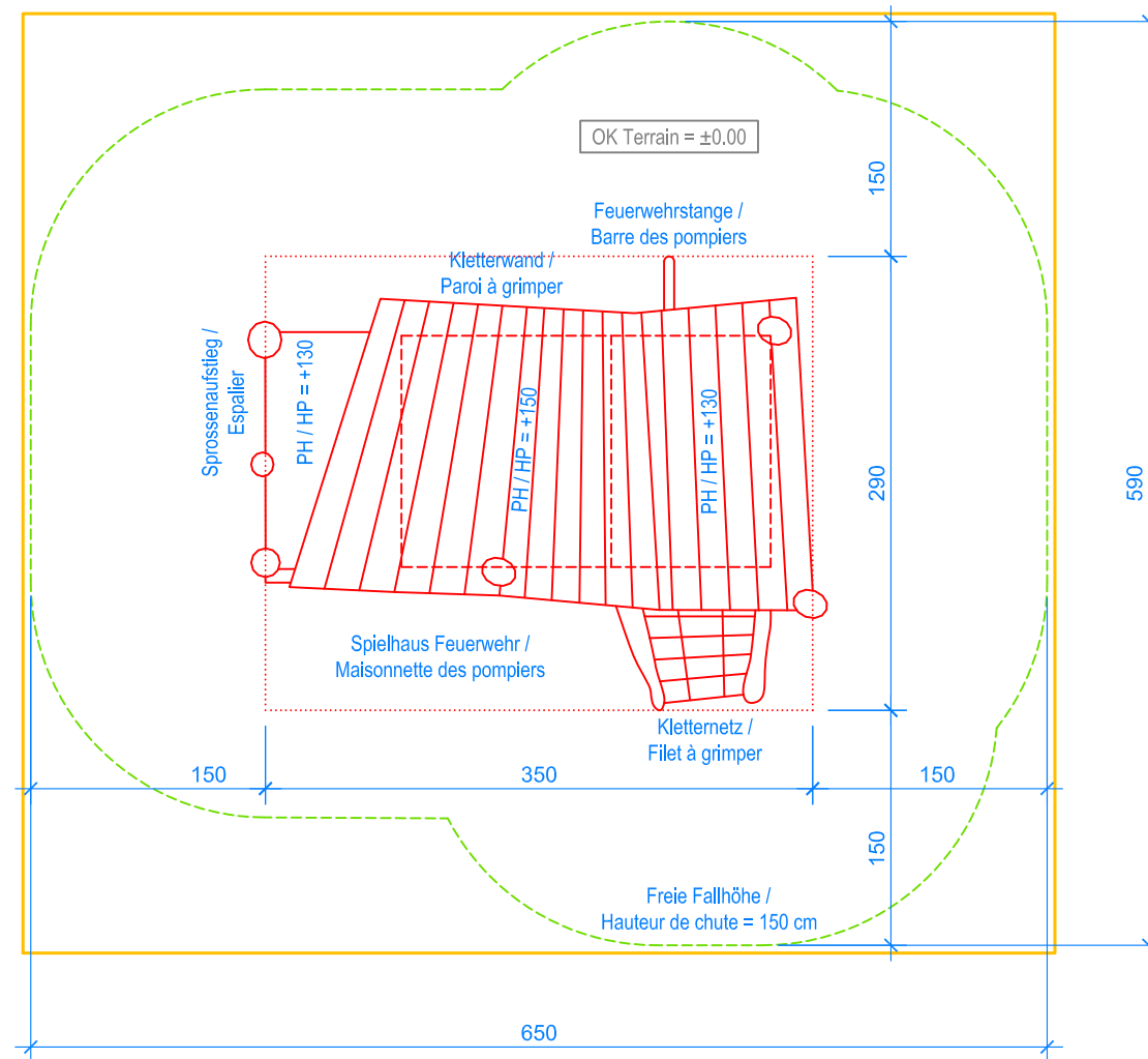
GRUNDRISS / PLAN 1:50
