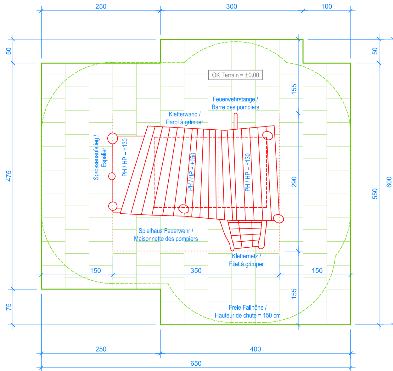
GRUNDRISS / PLAN 1:50
