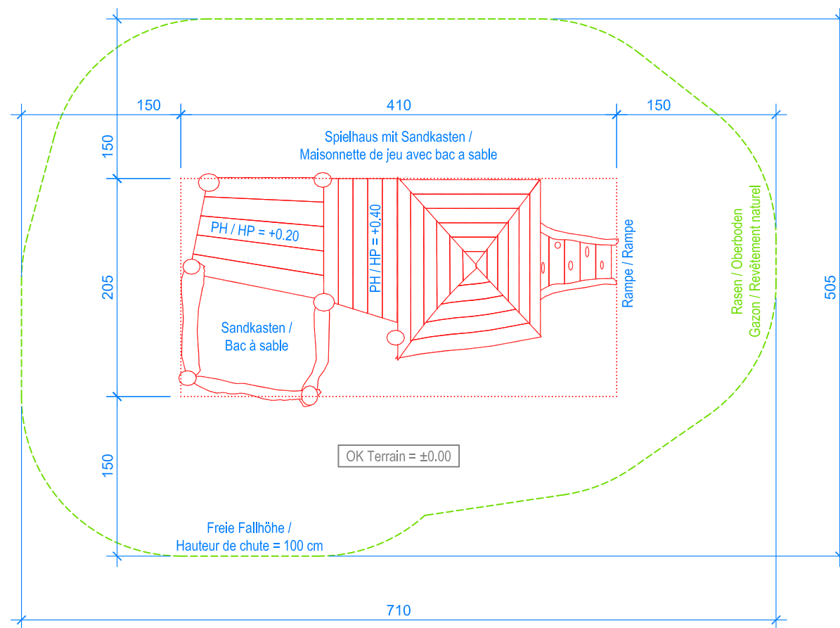
GRUNDRISS / PLAN 1:50
