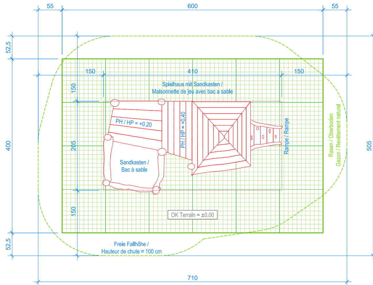
GRUNDRISS / PLAN 1:50
