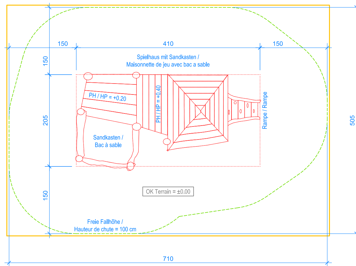
GRUNDRISS / PLAN 1:50
