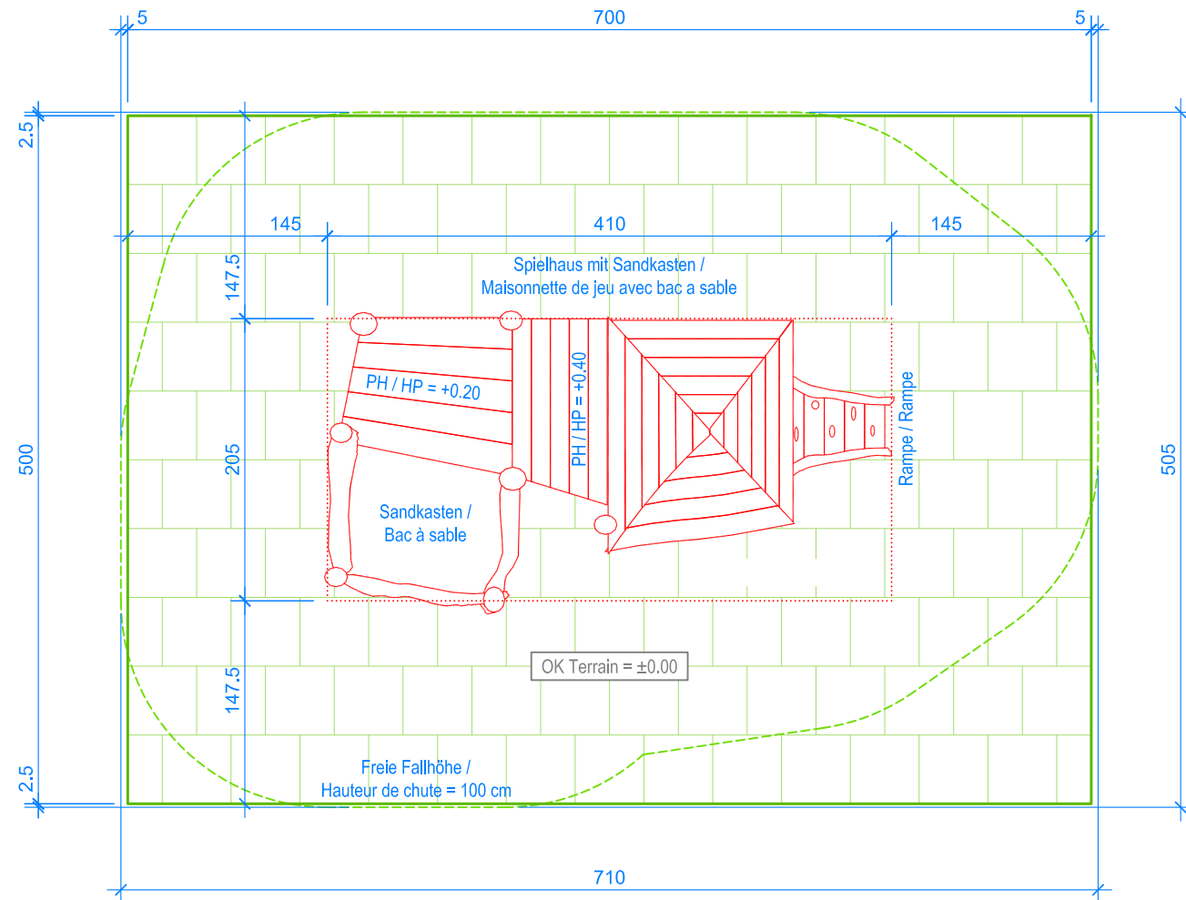
GRUNDRISS / PLAN 1:50
