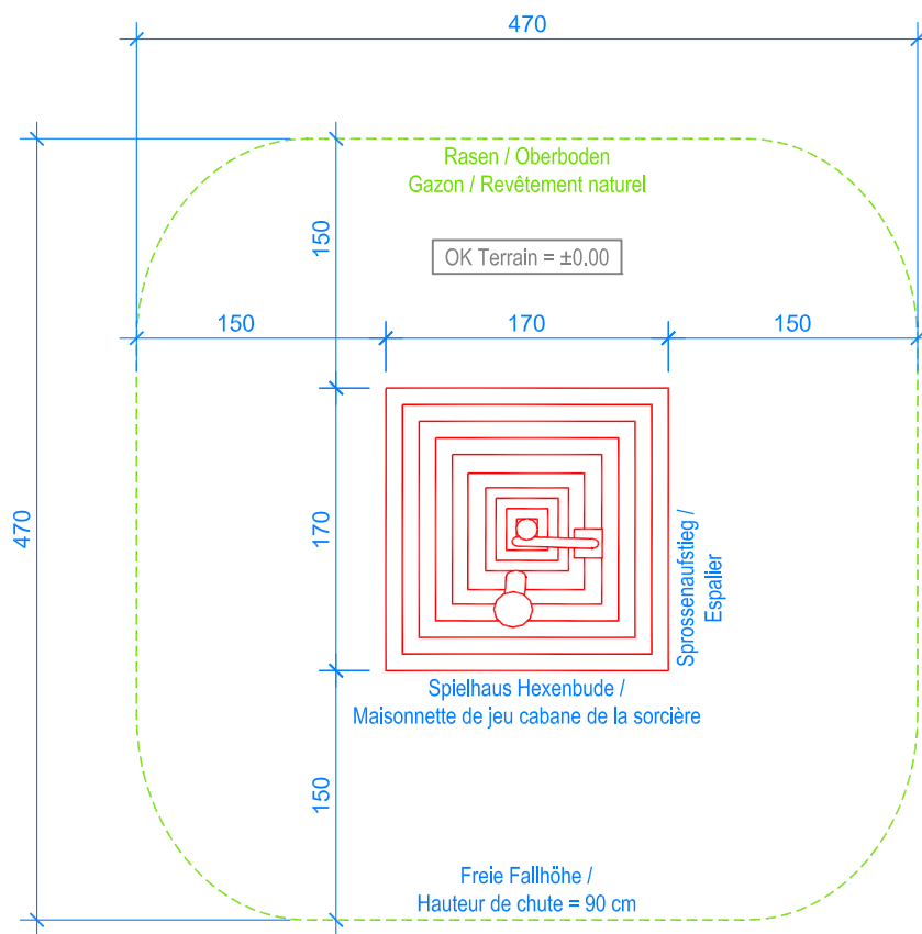
GRUNDRISS / PLAN 1:50
