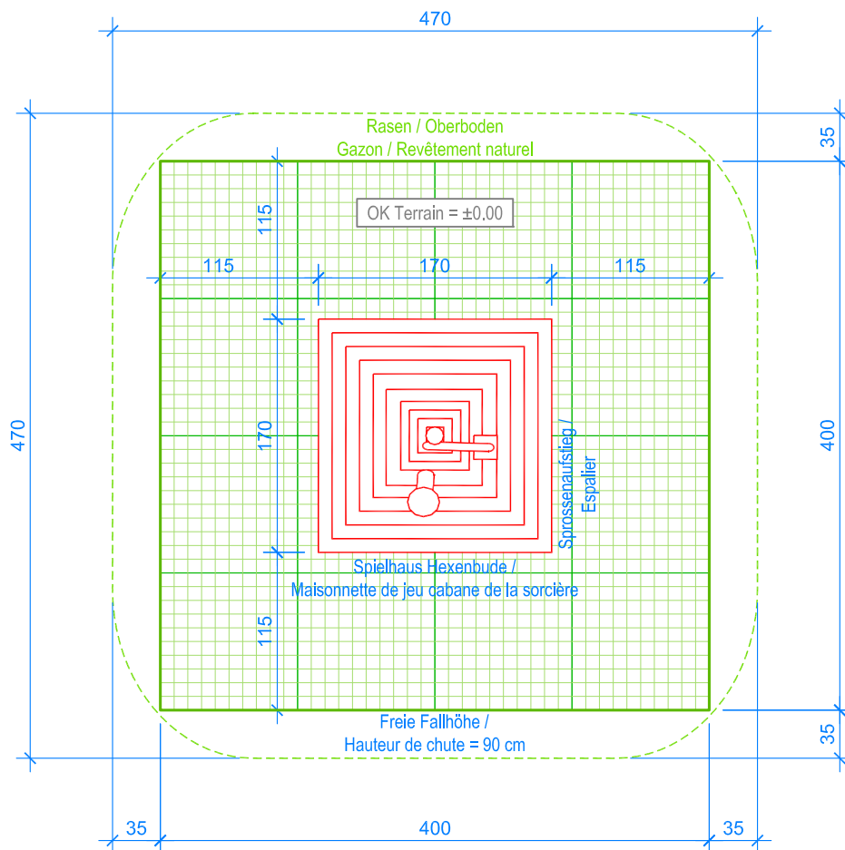
GRUNDRISS / PLAN 1:50
