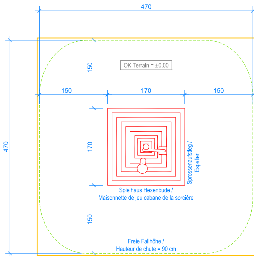
GRUNDRISS / PLAN 1:50
