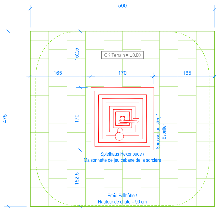
GRUNDRISS / PLAN 1:50
