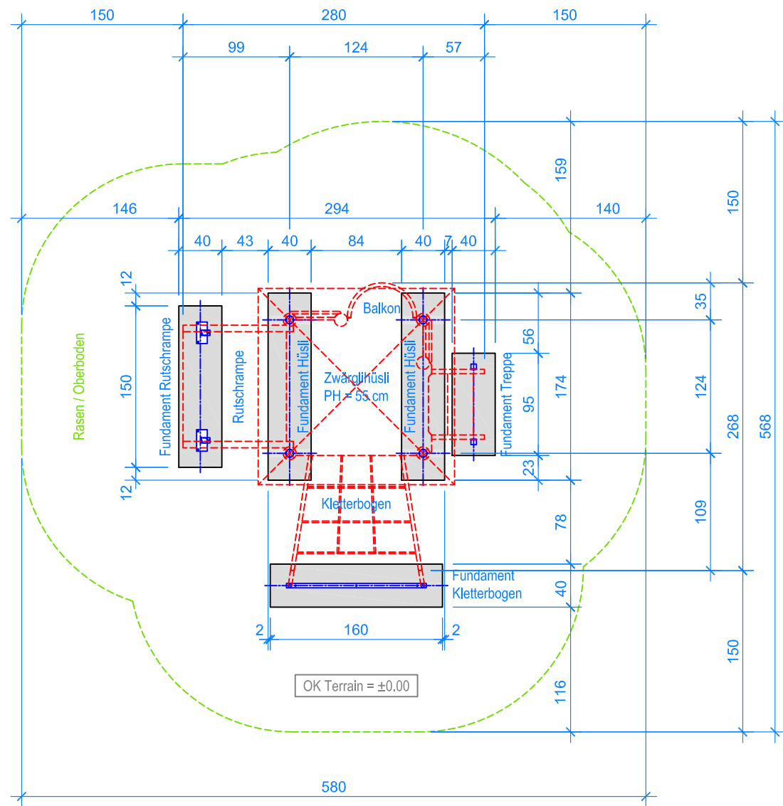
GRUNDRISS 1:50
