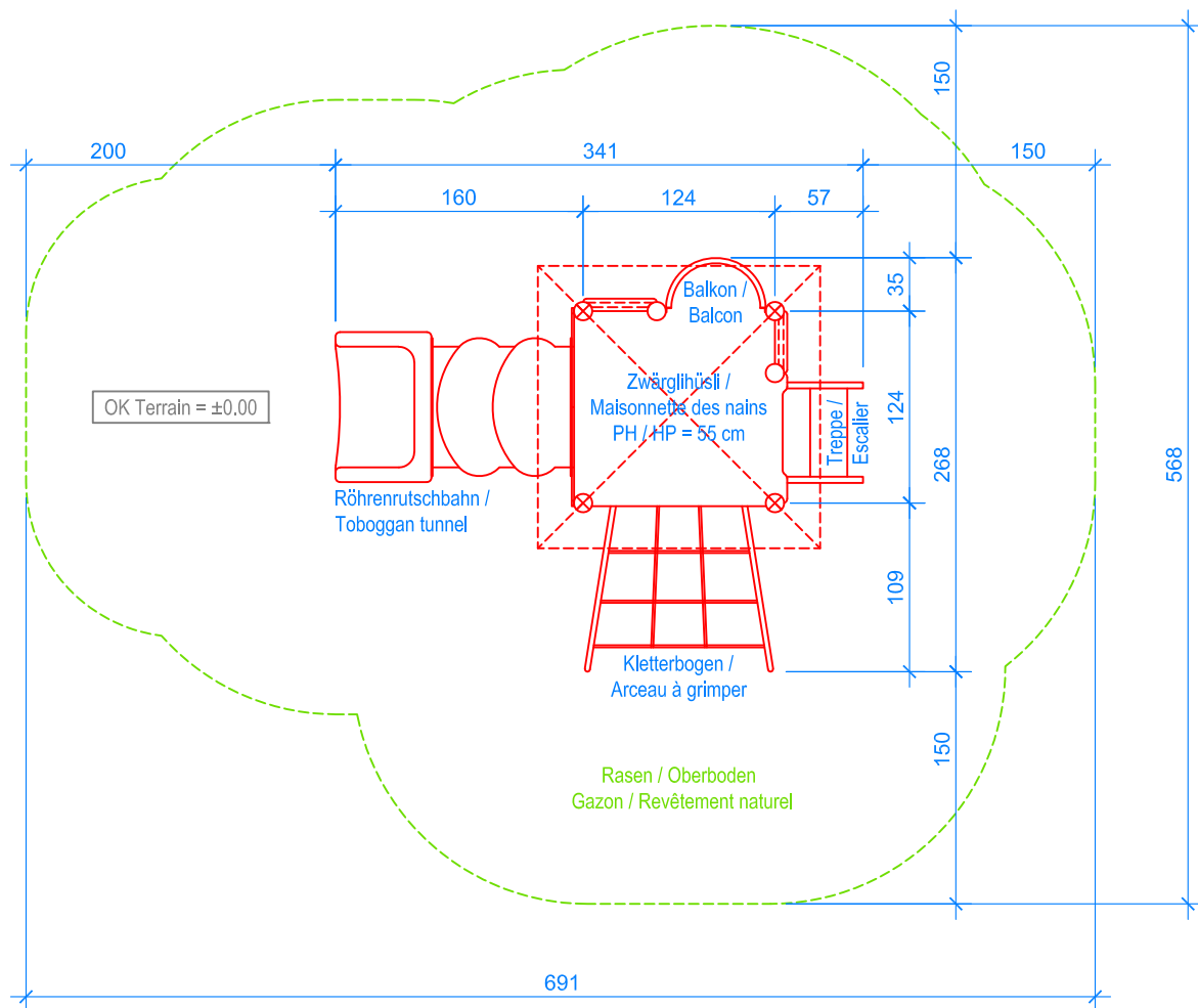
GRUNDRISS / PLAN 1:50
